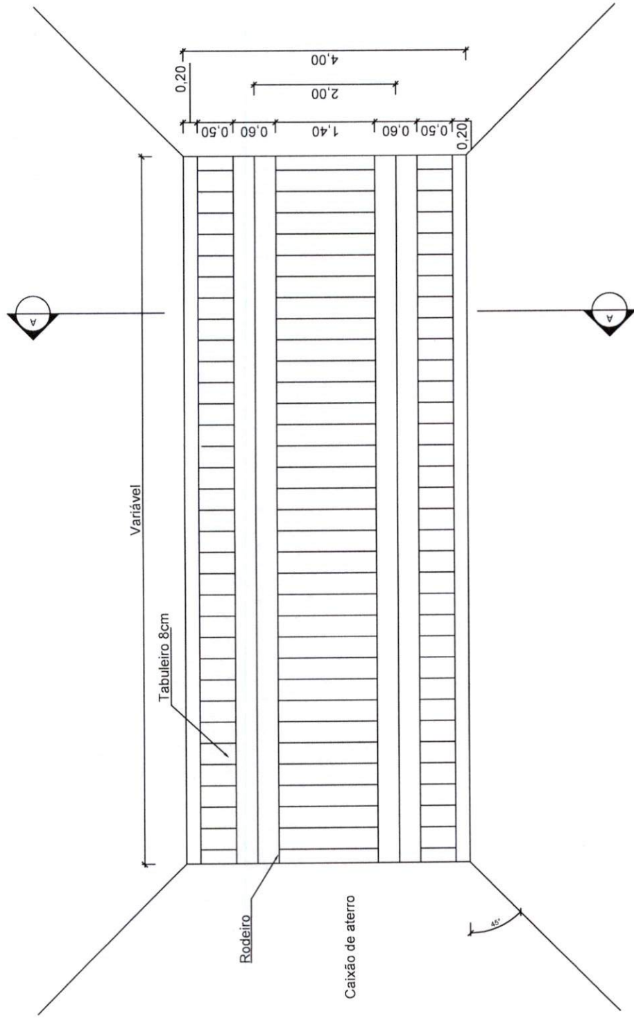
01 PLANTA BAIXA SEM ESCALA
