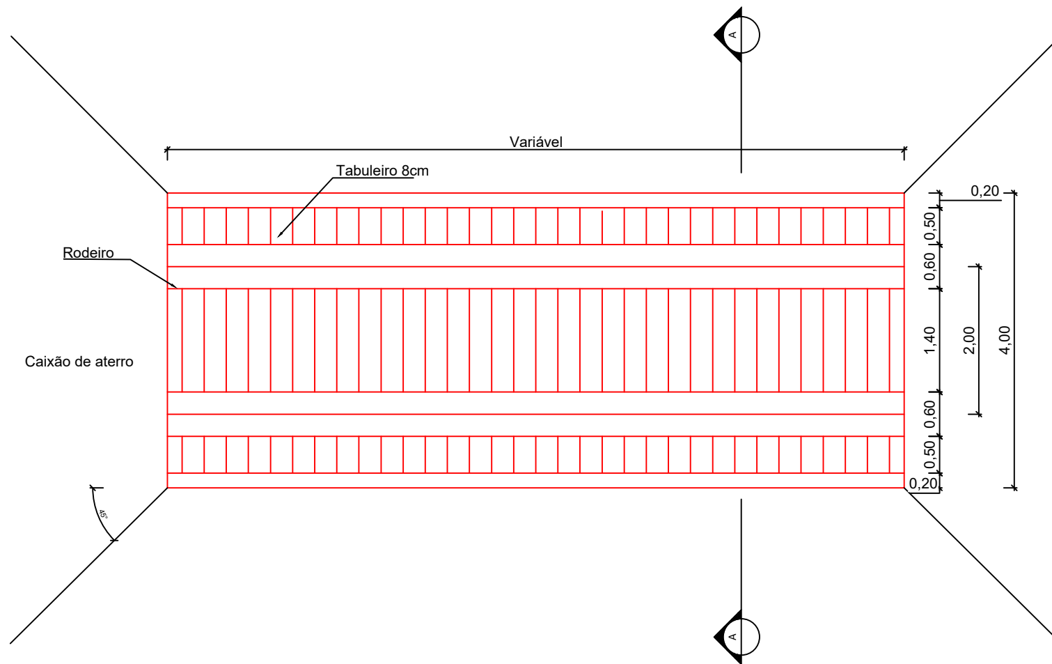
01 PLANTA BAIXA SEM ESCALA
